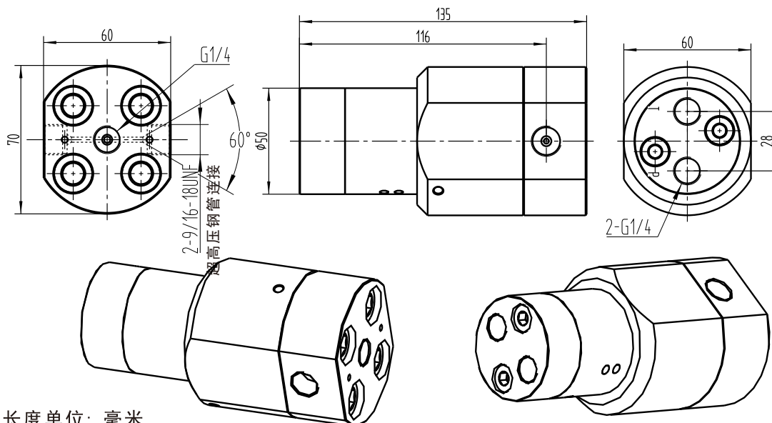
安装尺寸
